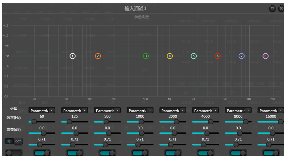
图 3.6 均衡器
